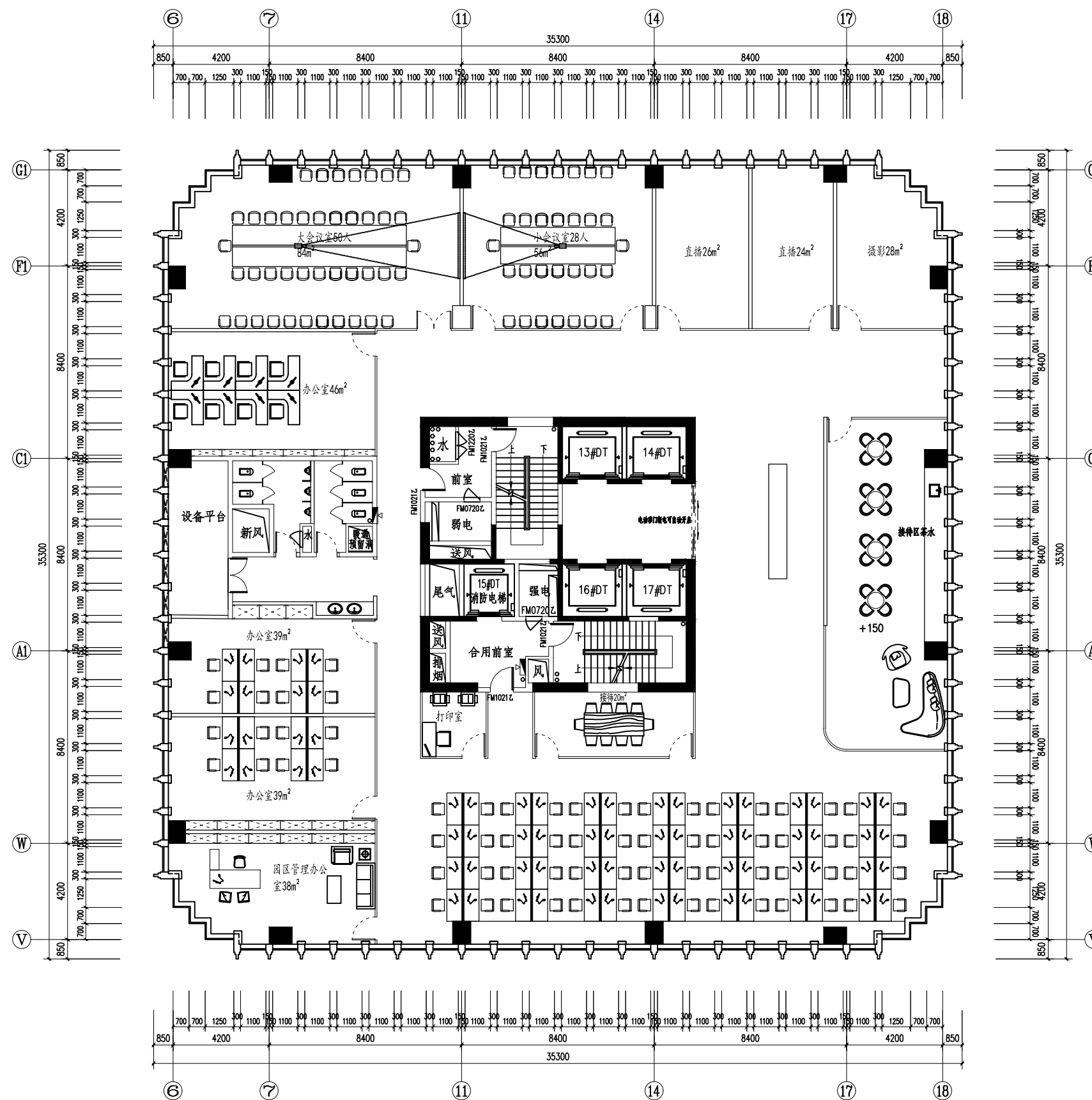
八层平面布置图 1:100
